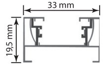
Шинасым қимасының габариттері
