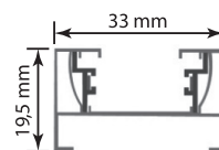
Габариты сечения шинопровода
