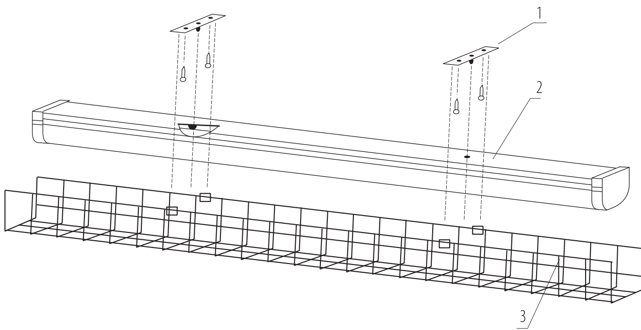
Рисунок 1. Схема монтажа защитной решётки
